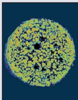
Distribución de magnesio en el interior de un cóndrulo del meteorito Allende.
